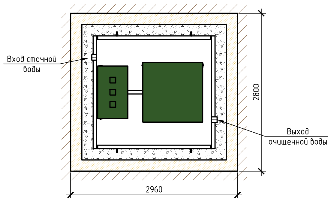
Вид сверху
