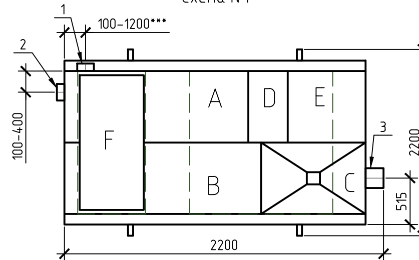
Схема №1
